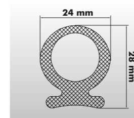
Fingerschutzprofil
