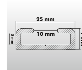
Aluminiumhalteleiste
